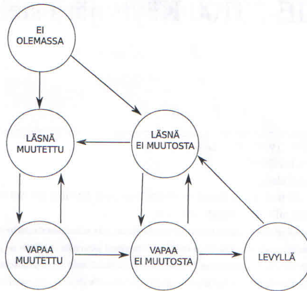
Kuva 1: Muistisivun tilamalli
