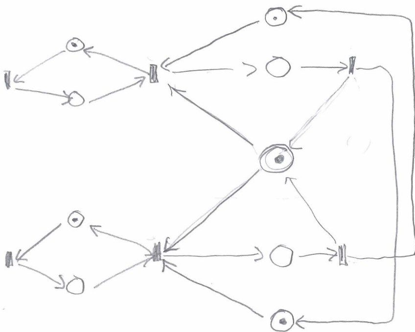
petri net
